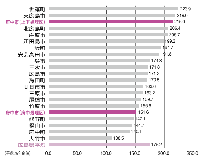
下水道の使用料単価 (円/m³)
