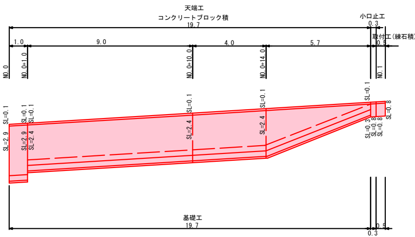
コンクリートブロック積展開図 S=1:100
