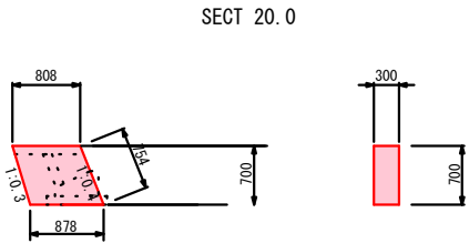
小口止工 S=1:50
