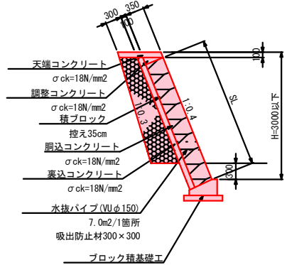
コンクリートブロック積工 S=1:50
