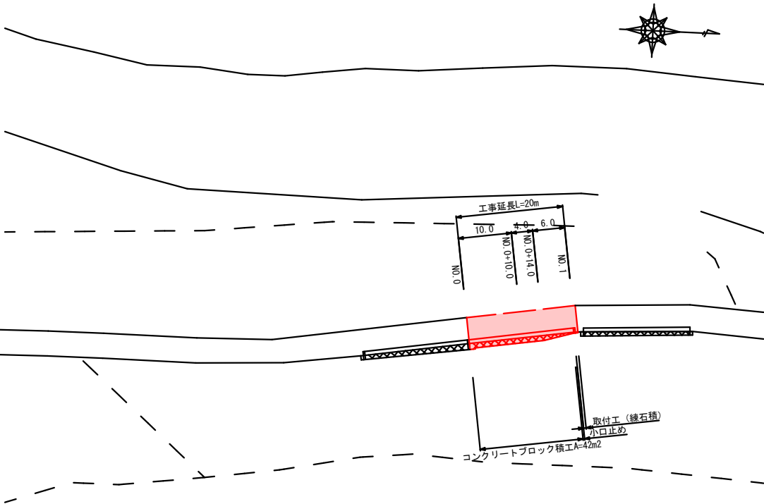
平面図 S=1:500
