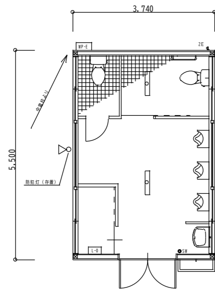
電気設備図 1/50
