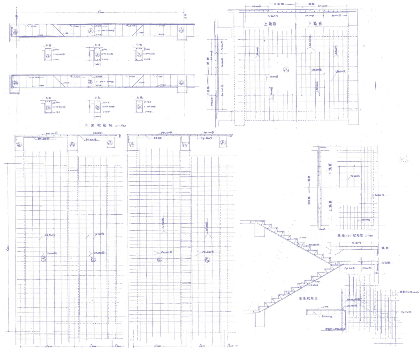
スラブ・階段配筋図 1/50
