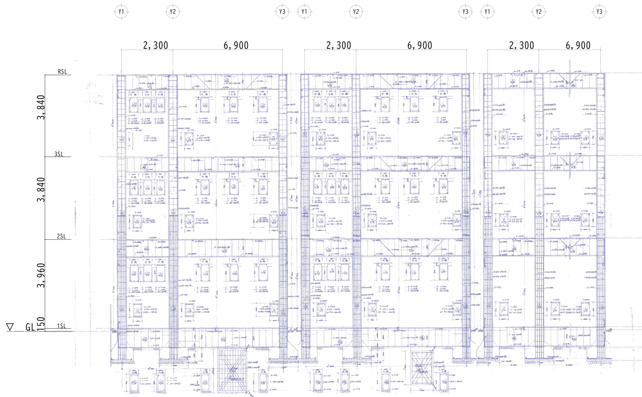
X1 通りラーメン配筋図
