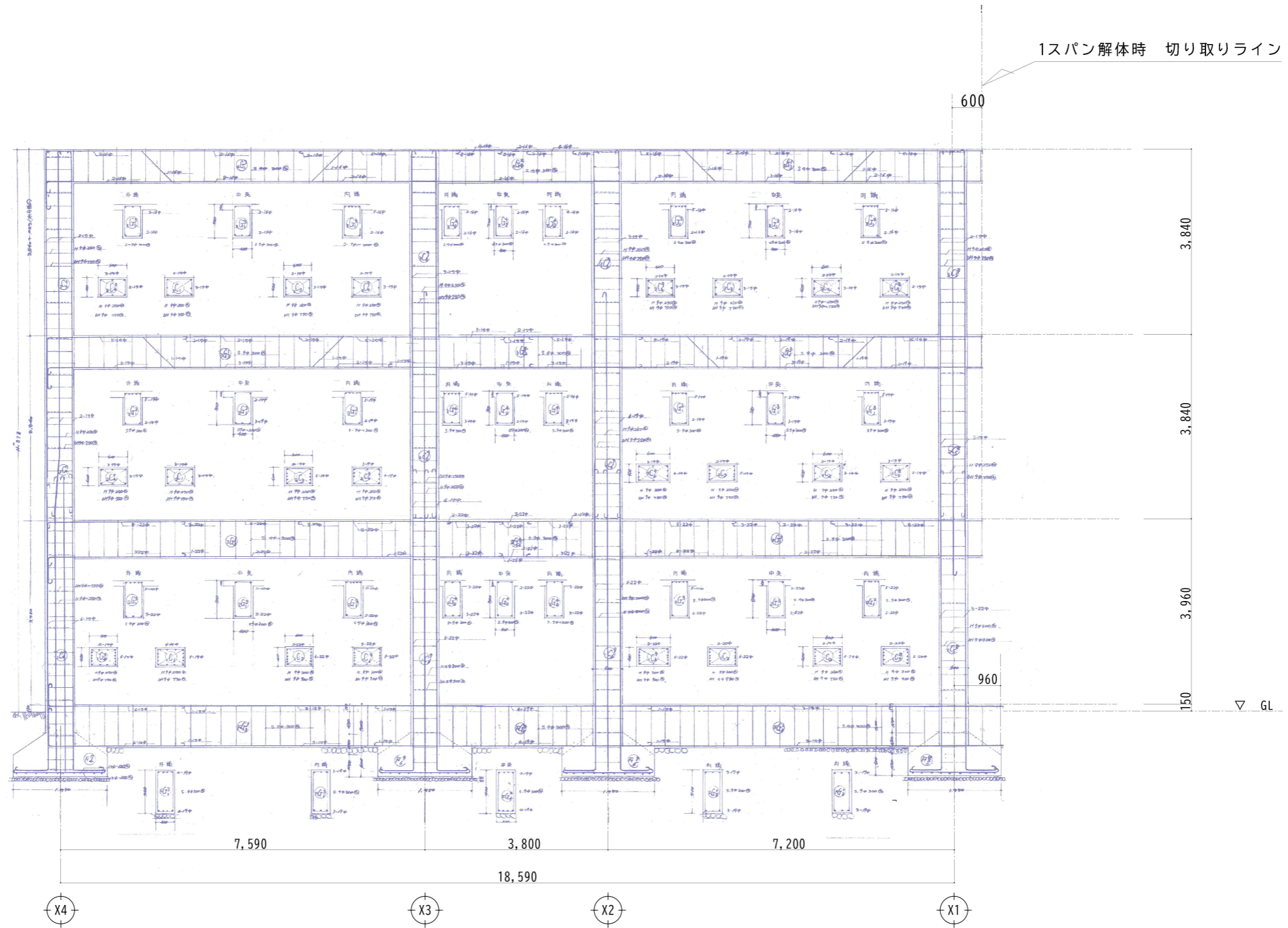
Y4 通り ラーメン配筋図 1/50
