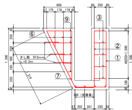
C-C断面
