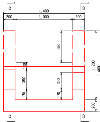
側面図 (C-C断面)
