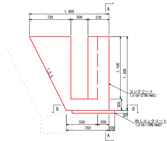
側面図 (B-B断面)
