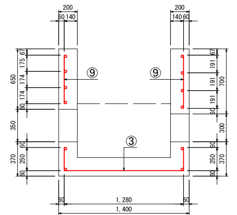
E-E断面
