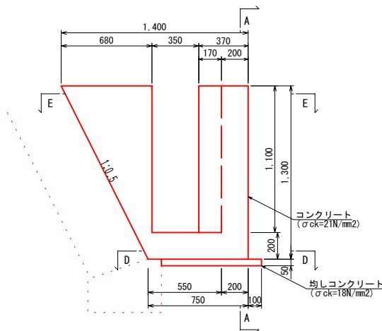
側面図 (C-C断面)
