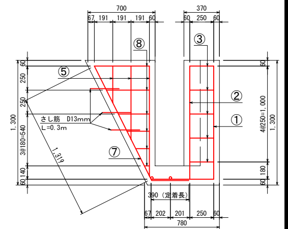
D-D断面
