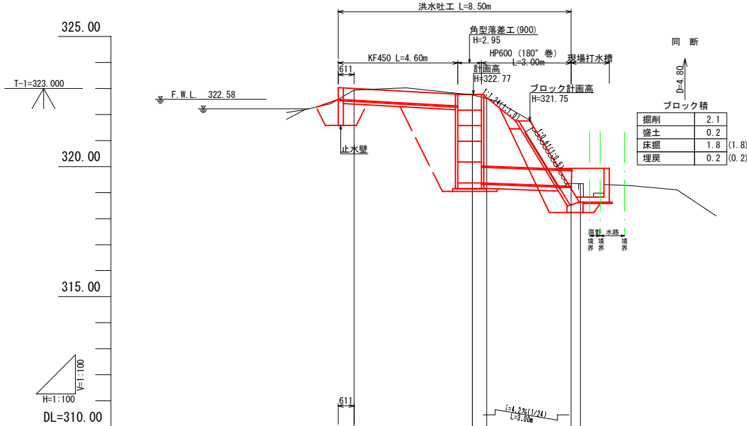
縦断面図
