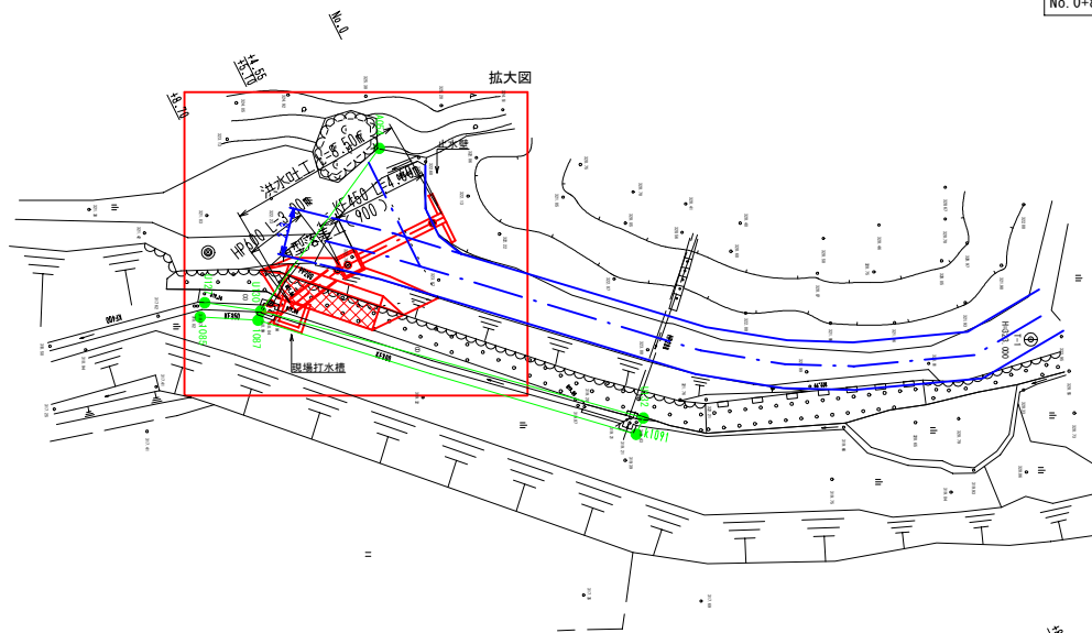
計画平面図
