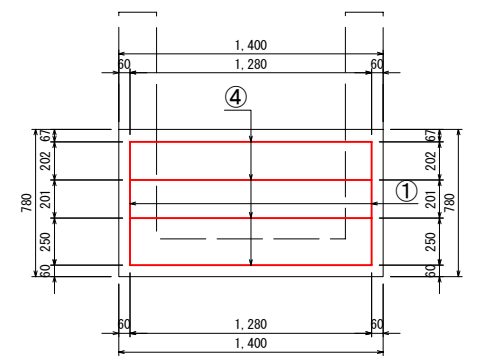
E-E断面
