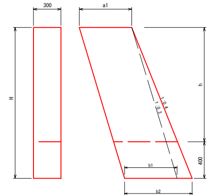
小口止工 S=1:20
