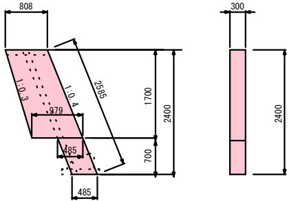
2号 小口止工 S=1:50
