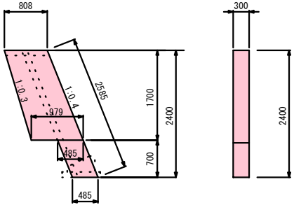
1号 小口止工 S=1:50
