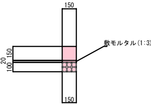
境界ブロック S=1:20
