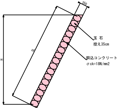
取付工（練石積） S=1:50
