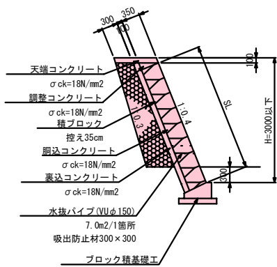
コンクリートブロック積工 S=1:50
