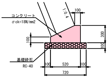
ブロック積基礎工 S=1:20
