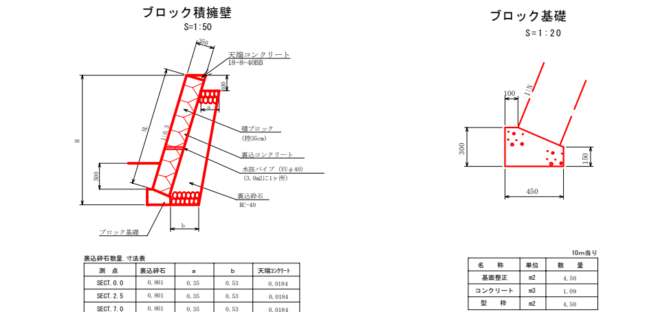
構造図
