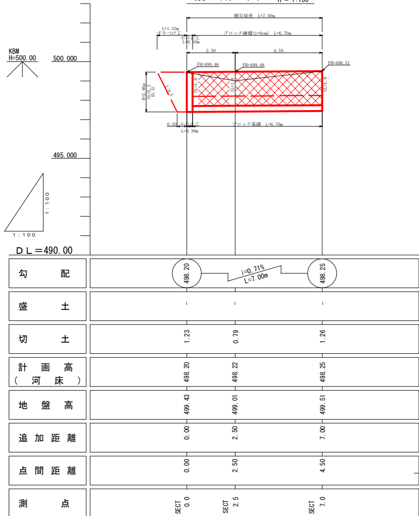
縦断面図 V = 1:100 H = 1:100
