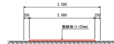
仮設道路 (敷鉄板)
