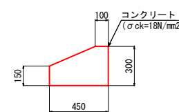
ブロック基礎
