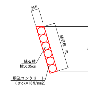
すりつけ工
