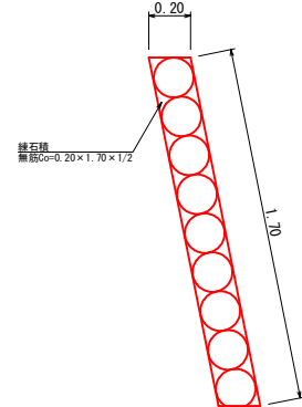
構造物取壊し工
