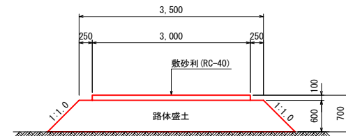
仮設道路 (盛土)
