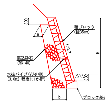
ブロック練積 (t=0cm)
