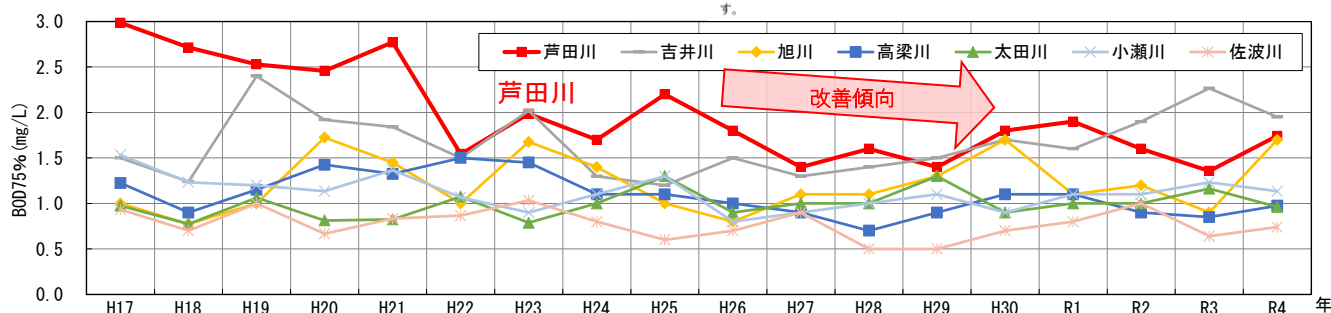
【図5：BOD75%値の経年変化(山陽側河川を表示)】
