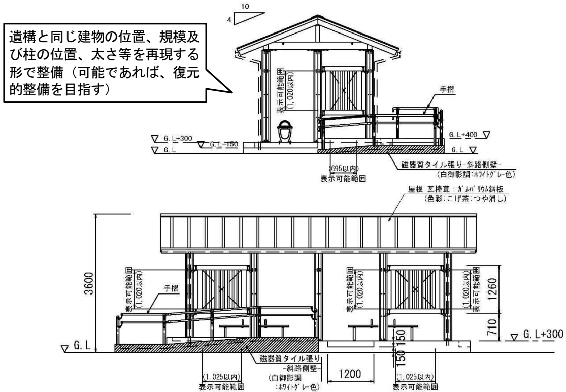
図 5-20 ガイダンス機能を有する休憩施設・あずまやのイメージ（参考図）
