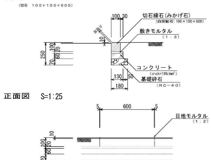
図 5-11 建物界線の平面表示の方法（参考図）
