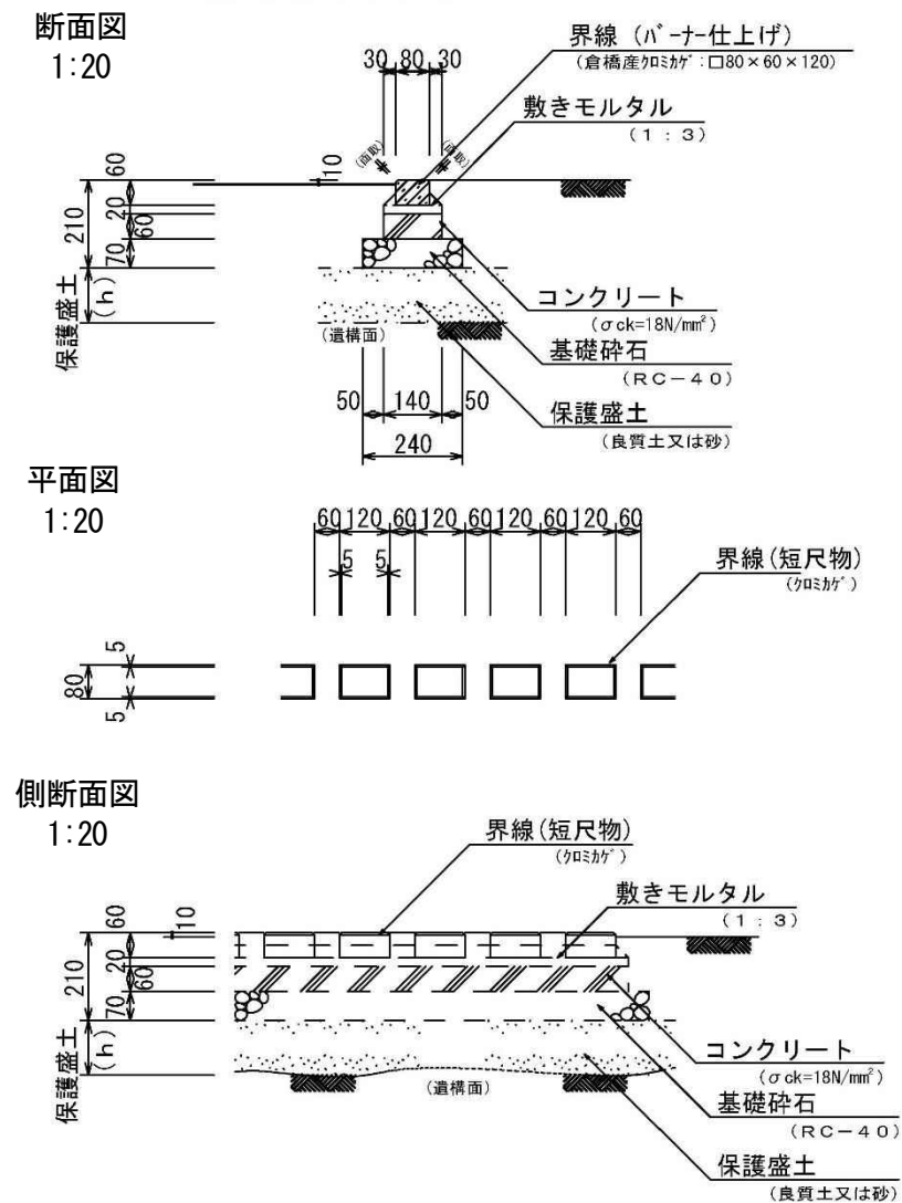
図 5-9 建物界線の平面表示の方法 (短尺：参考図)
