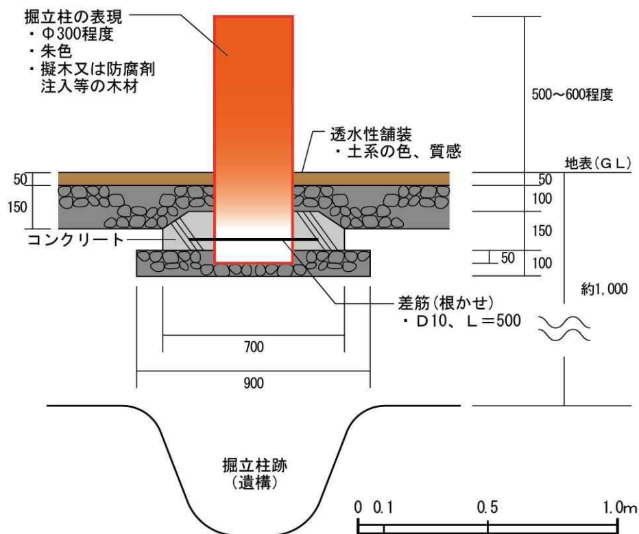
図 5-7 掘立柱の立体表示
