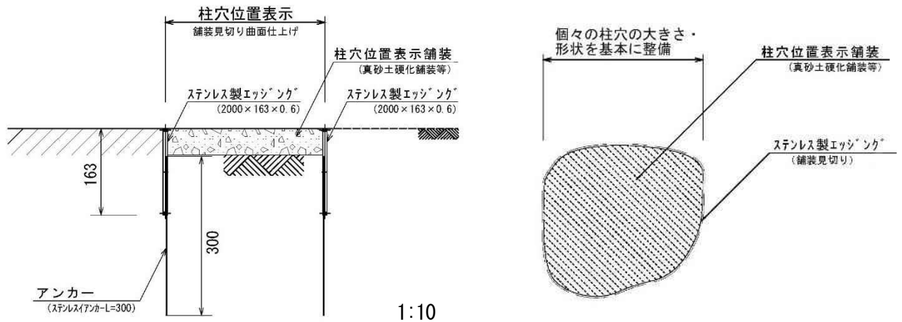
図 5-8 柱穴の平面表示の方法 (参考図)
