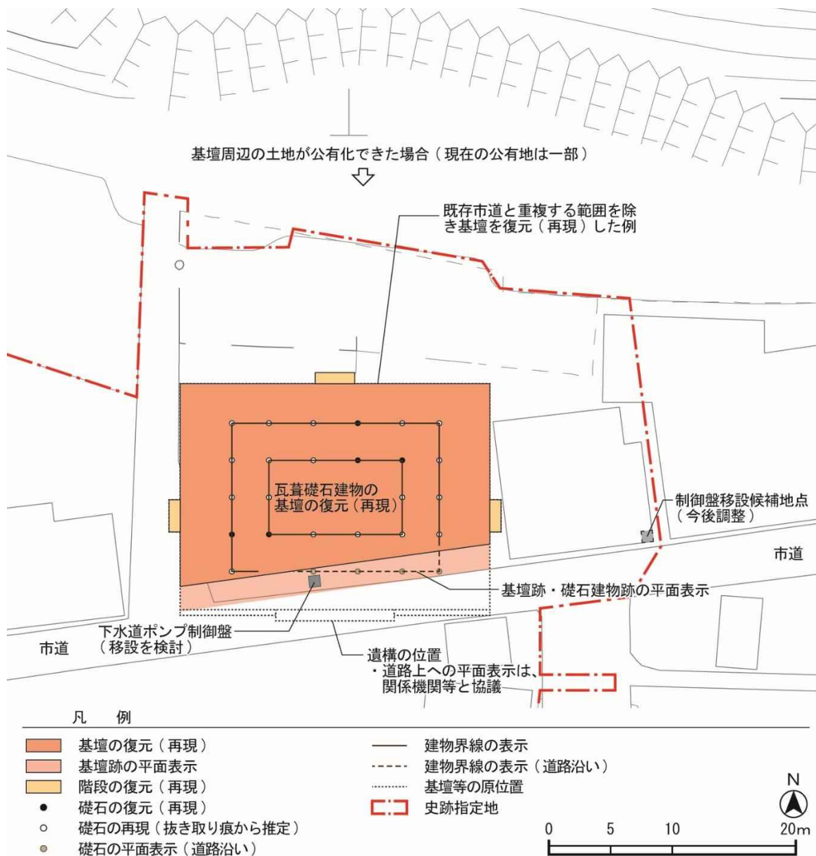
図 5-12 基壇の一部復元的整備及び礎石建物跡の表示（原位置での整備）
