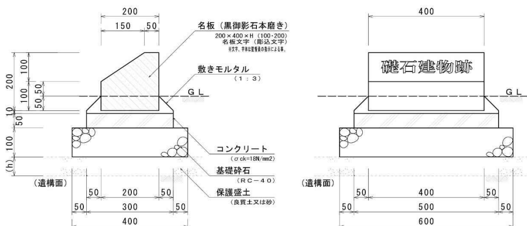
図5-22 名称表示板（立ち上がり型）の整備例（参考図）
