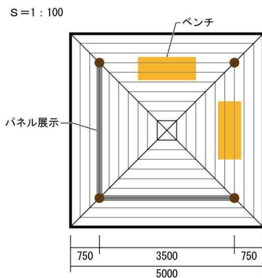
図 5-25 ガイダンス機能を有する休憩施設(あずまや)の平面イメージ(屋根も表示)
