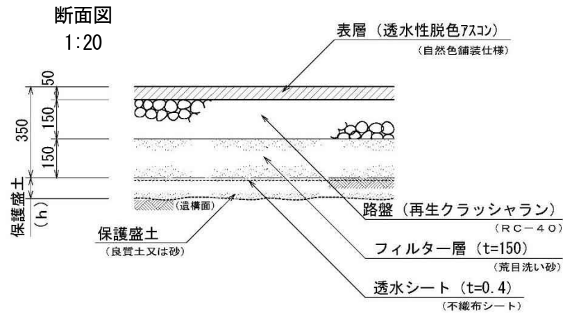
図 5-10 建物跡（範囲）の平面表示の方法（断面図：参考図）
