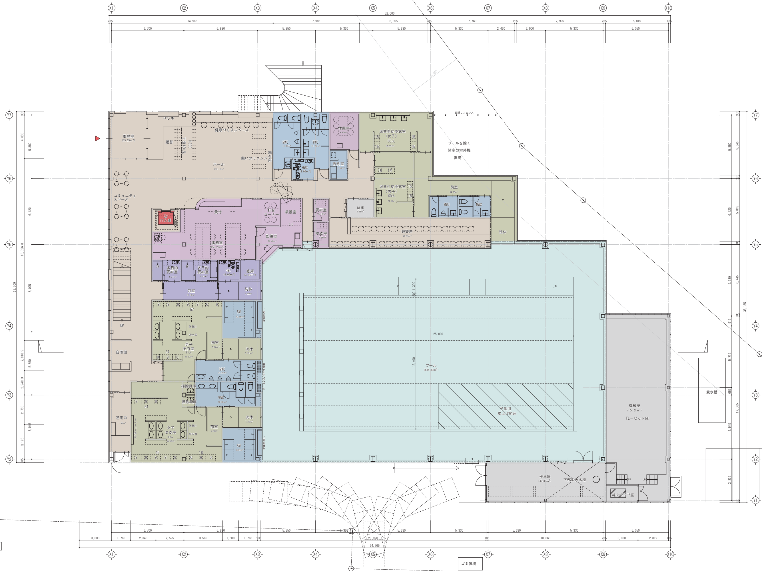
1階平面図
